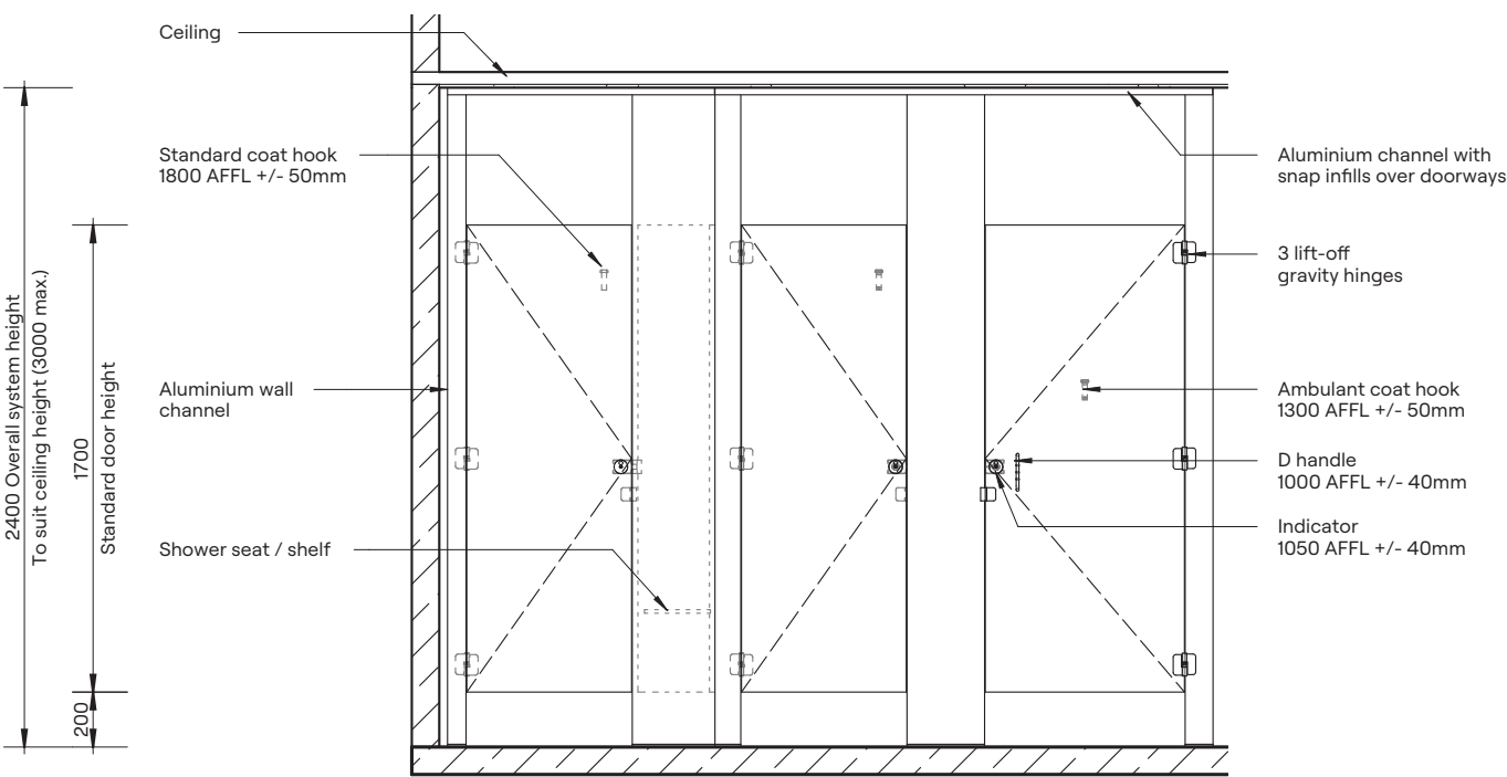
Elevation
