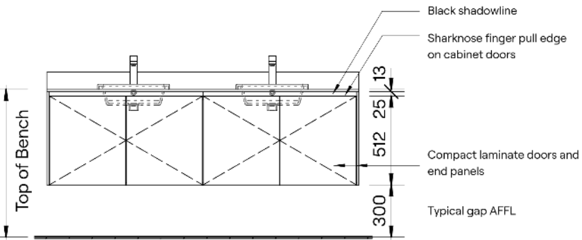
Elevation
