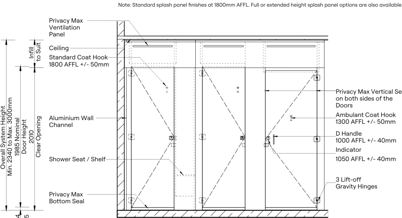
Elevation
