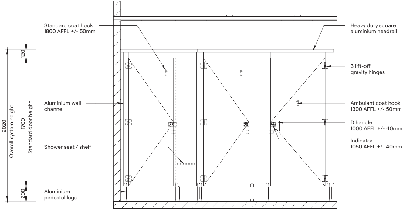
Elevation
