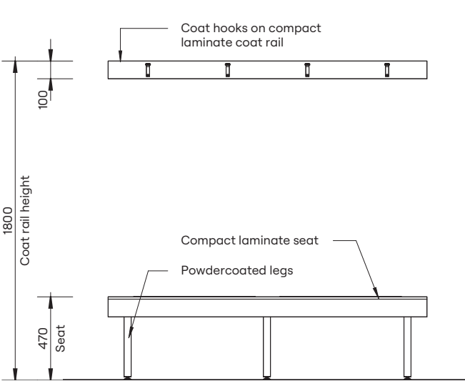
Elevation
