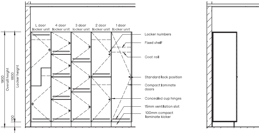
Elevation
