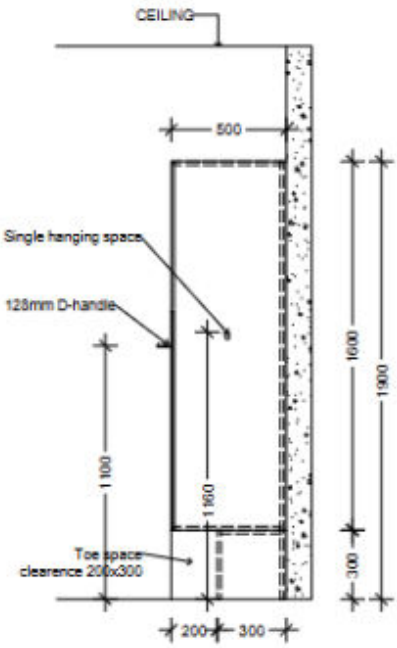
Elevation B
