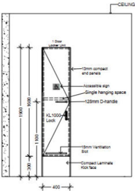
Elevation A
