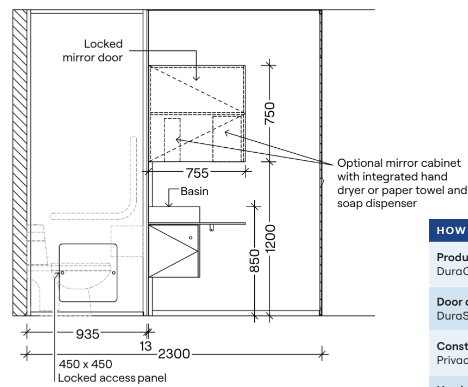
Elevation B
