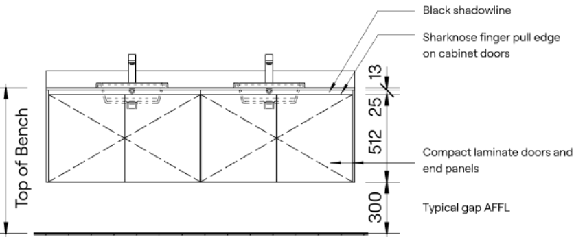
Elevation
